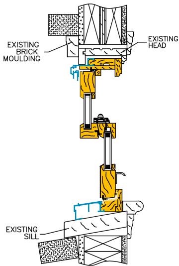
CLAD DOUBLE HUNG DHC250 (EC200)
